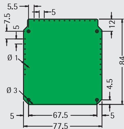
Leiterkartenabmessung
